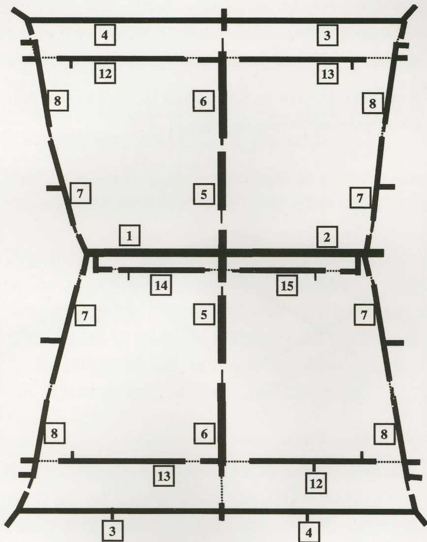
Figura 3. Disposizione paleria tetto
